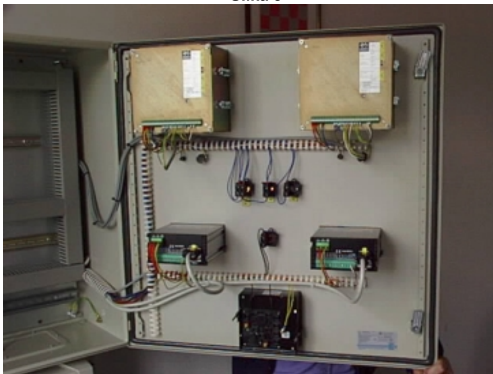
Unutrašnjost upravljačkog ormara
